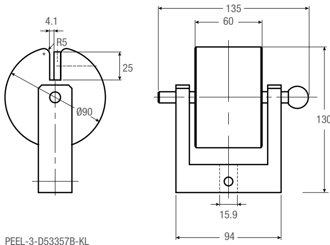
PEEL-3-D53357B-KL
