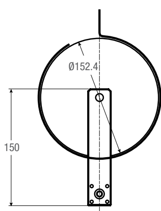
PEEL-3-IS06133L
