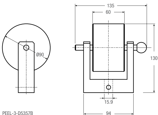
PEEL-3-D53357B
